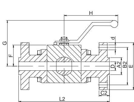
Фланцевое соединение
